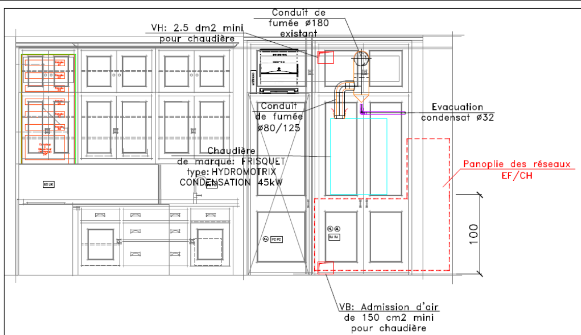
COUPE AA – Ech: 1/20
