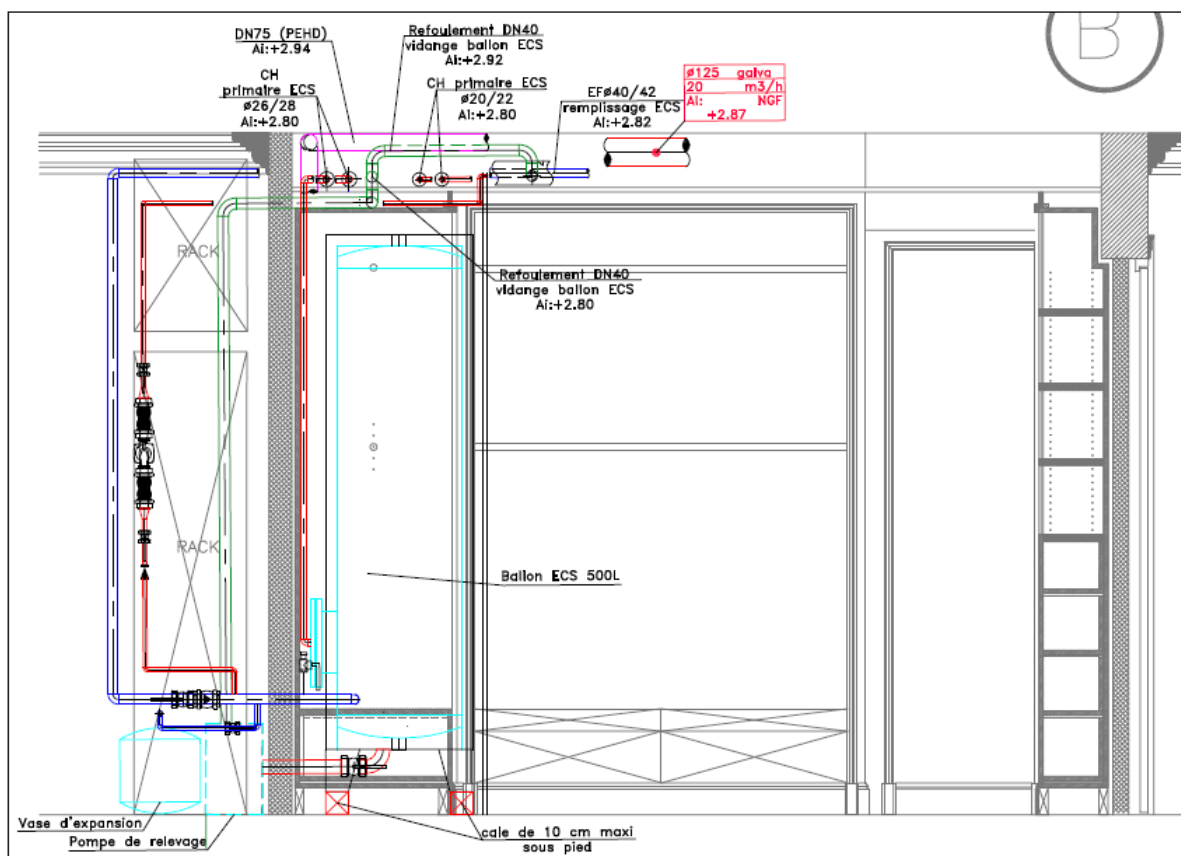
COUPE BB – Ech: 1/20
